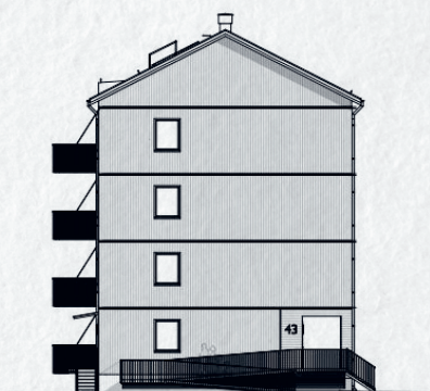
FASAD GAVEL MOT SÖDER
